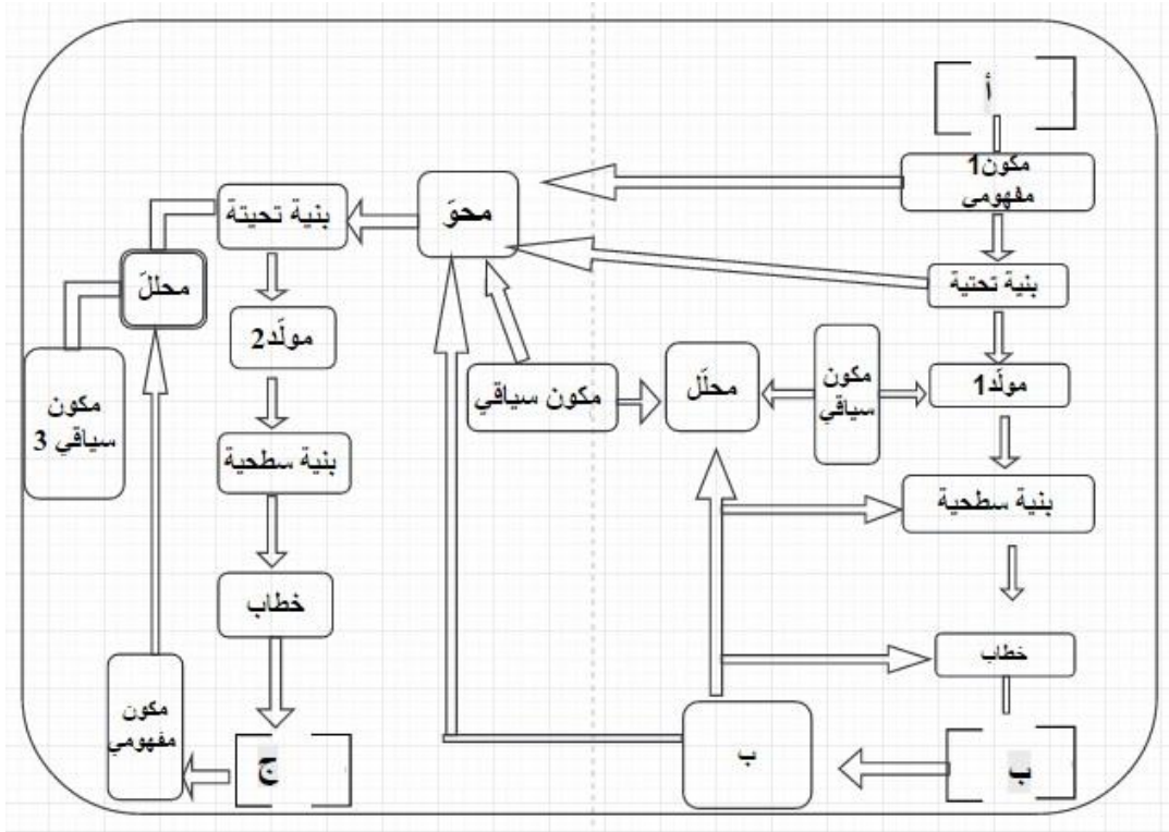
شكل (15): آلية إشتغال نموذج نحو الطبقات القالي الموسع
