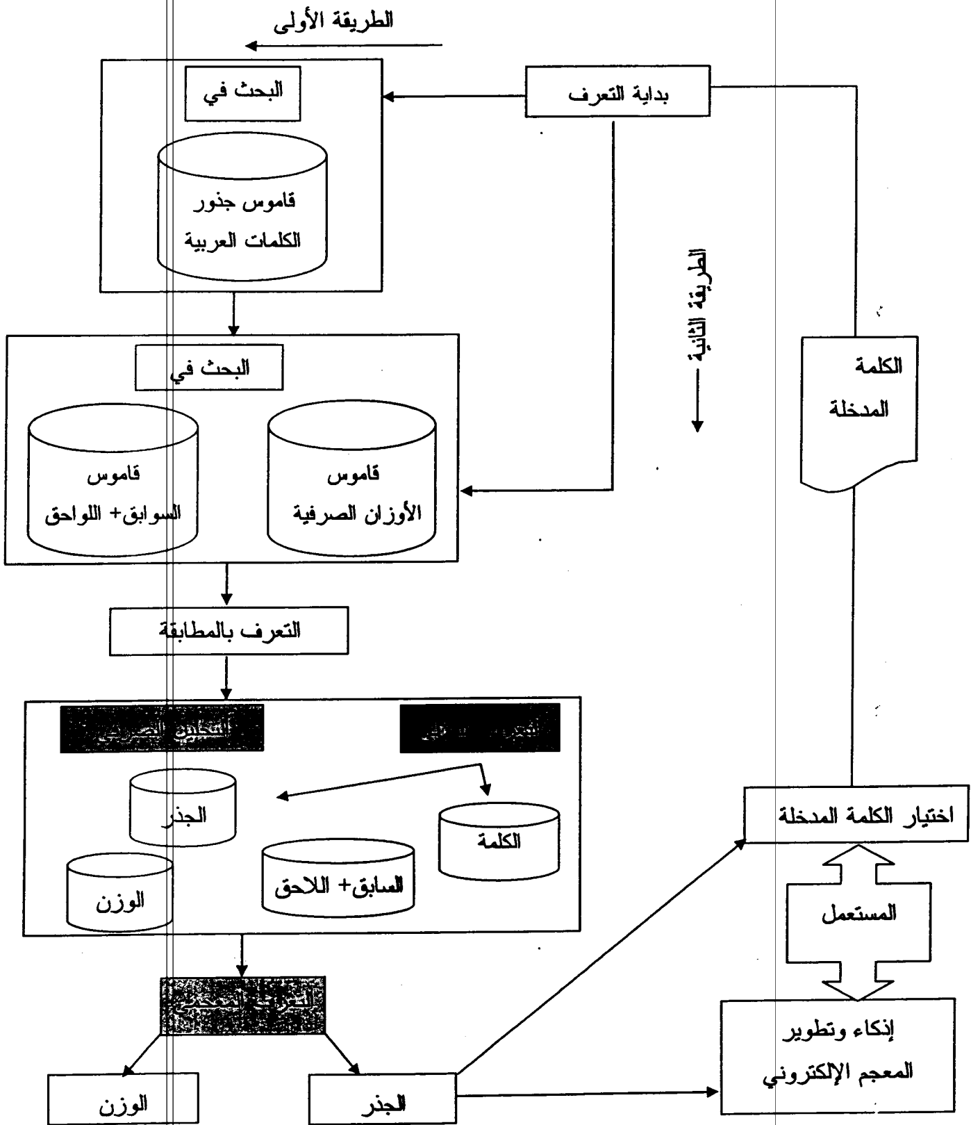
الشكل رقم 25: آلية التعرف على الكلمات العربية عن طريق استخراج الجذر والوزن المناسبين في المعجم الإلكتروني للمعالجة الآلية للغة العربية
