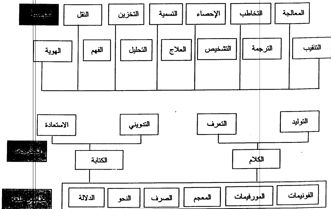
الشكل رقم 04: المنظومة المعرفية لبرمجة اللغة الطبيعية.
